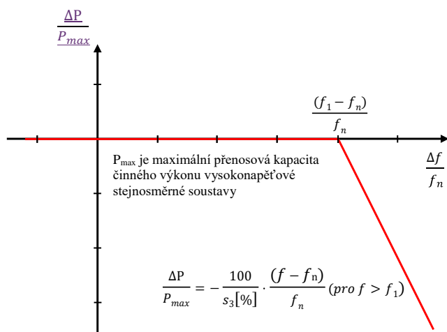
Obr. 4: Schopnost frekvenční odezvy činného výkonu u vysokonapětových stejnosměrných soustav v omezeném frekvenčně závislém režimu při nadfrekvenci. \Delta P je změna činného výkonu na výstupu z vysokonapětové stejnosměrné soustavy a v závislosti na provozních podmínkách buď snížení importovaného výkonu, nebo zvýšení exportovaného výkonu. f_n je jmenovitá frekvence střídavé soustavy nebo soustav, ke které (kterým) je vysokonapětová stejnosměrná soustava připojena, a \Delta f je změna frekvence střídavé
