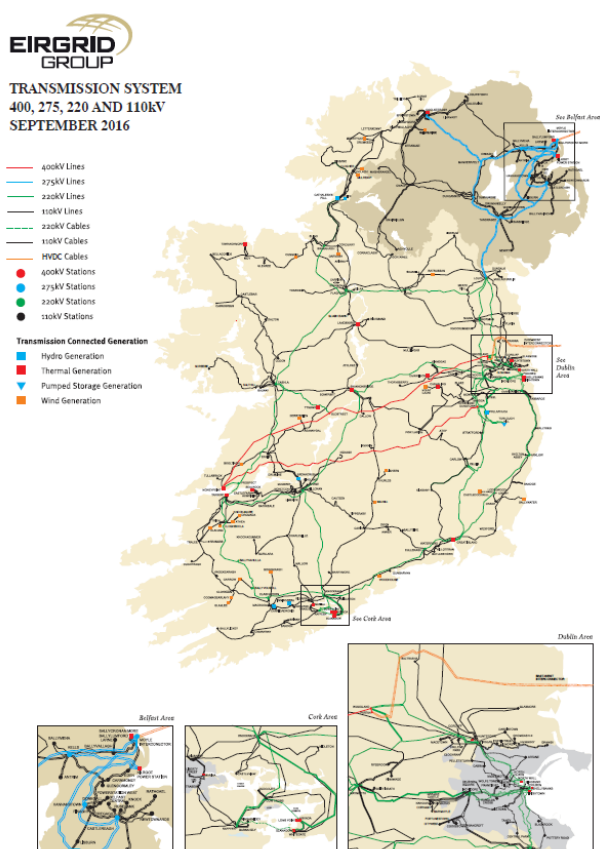
Obrázek 8: Mapa přenosové soustavy Irska a Severního Irska
