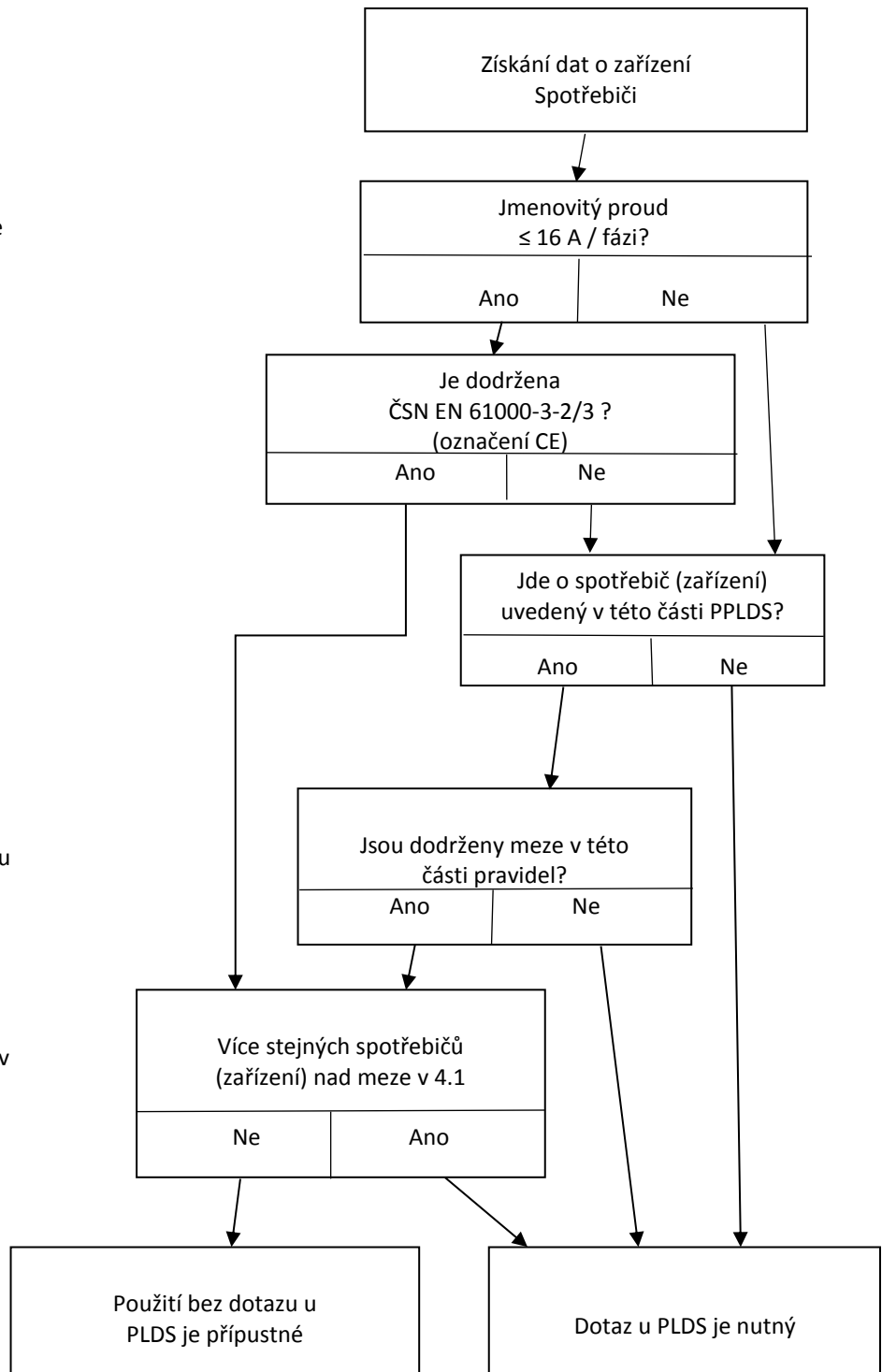
Obr. 1 Schéma po posuzování přístrojů/zařízení se zřetelem na elektromagnetickou kompatibilitu (EMC)
