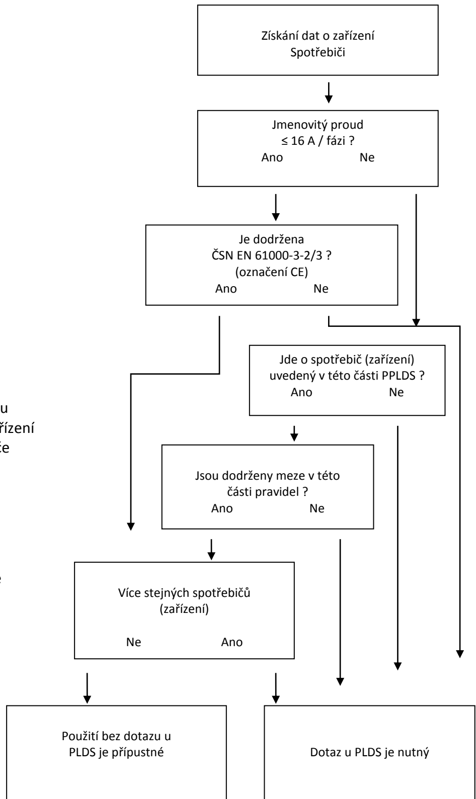
Obr. 1 Schéma po posuzování přístrojů/zařízení se zřetelem na elektromagnetickou kompatibilitu (EMC)
